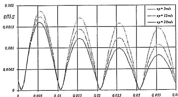
Rys. 9. Konduktancja wyładowania w funkcji czasu dla 3 prędkości gazu- wyniki numeryczne
