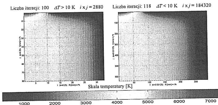
Rys. 13. Wynik symulacji numerycznej rozkładu temperatury w komorze wyładowczej reaktora ze ślizgającym się wyładowaniem łukowym
