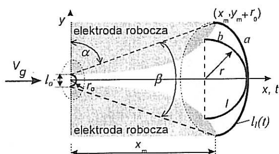
Rys. 8. Geometria elektrod z założonym kształtem kolumny ślizgającego się wyładowania łukowego: a – łuk oparty na kącie rozchylenia elektrod \beta
