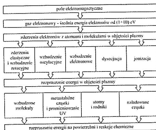
Rys. 1. Przemiany energii i zjawiska w plazmie Fig. 1. Energy conversion and phenomena in plasma
